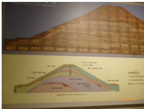
4. 狭山池堤の断面説明図
